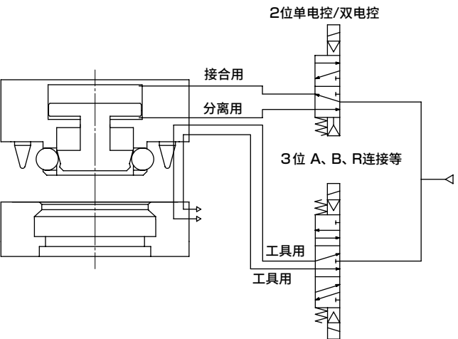
标准 推荐气动回路图
