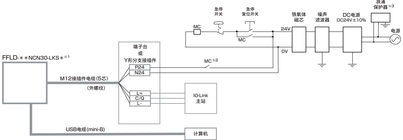
接线图
