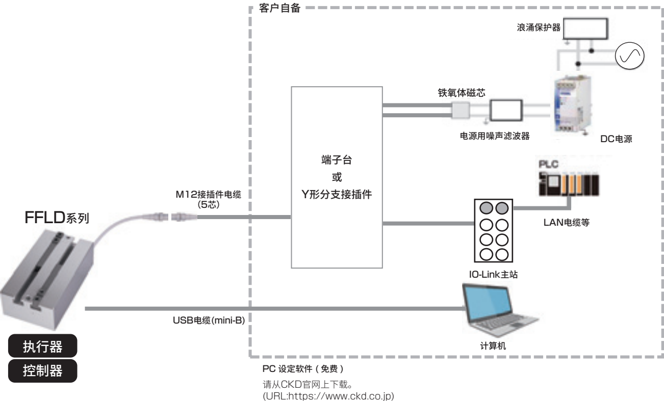
接线图
