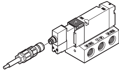
直线电缆型 (R3)
