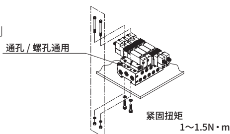
安装方法 M4G2・3系列
