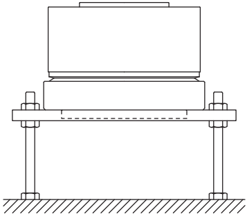
(图4) 安装刚性: 低
