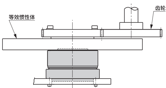
[图5] 等效惯性体安装示例3
