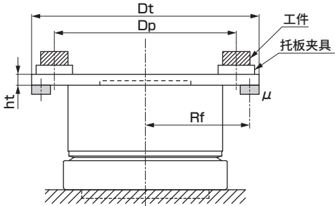
(图1) 负载条件
