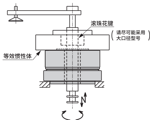
[图5] 等效惯性体安装示例3
