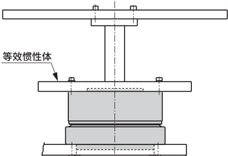
[图3] 等效惯性体安装示例1
