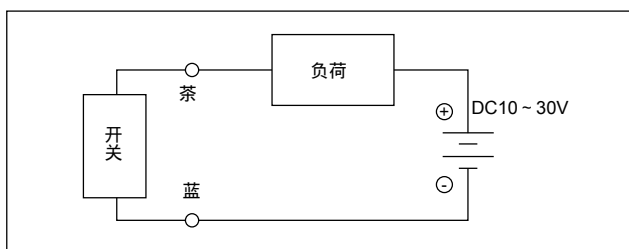
导线的连接
