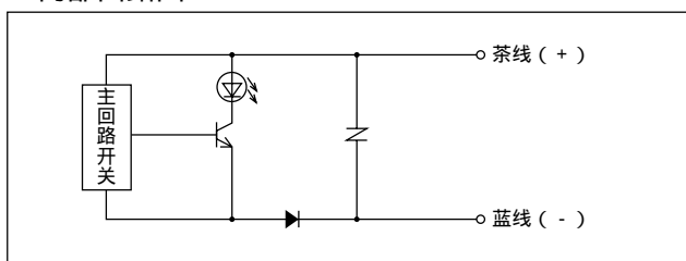
内部回路图
