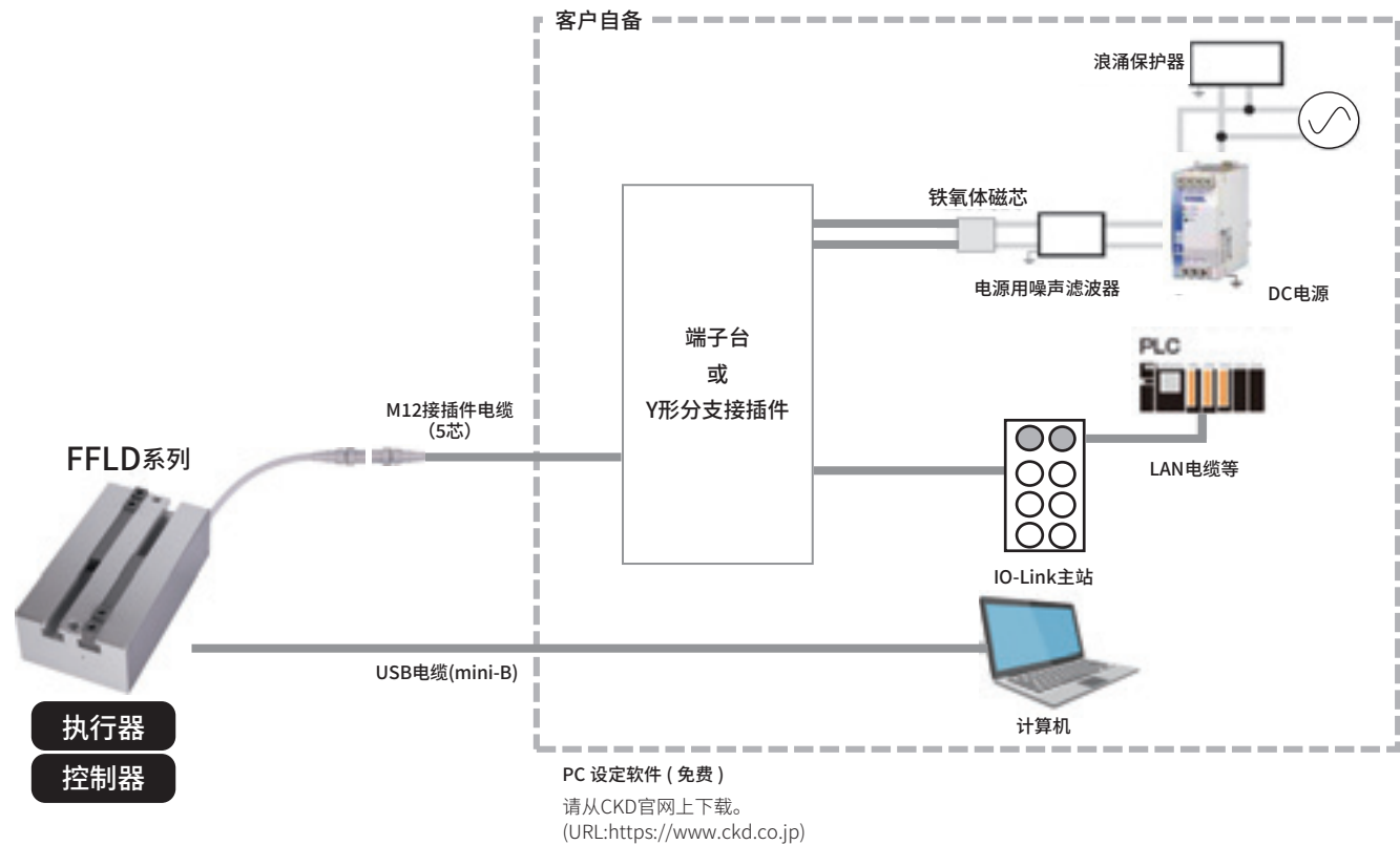
接线图
