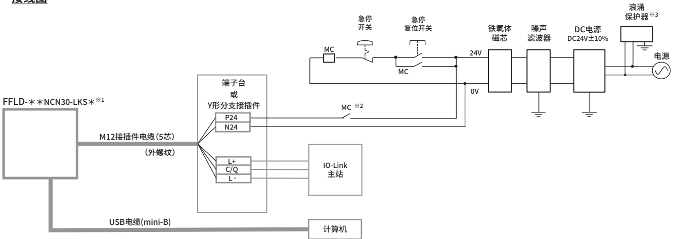
接线图
