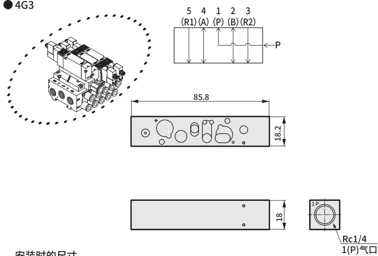
安装时的尺寸
