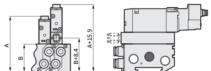
安装时的尺寸
