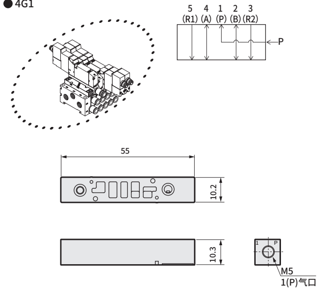
安装时的尺寸
