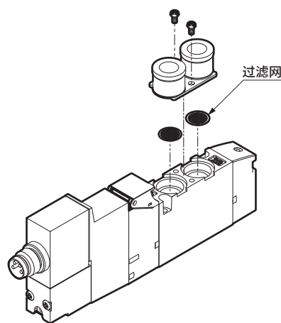
A・B口过滤网选择项组装示例
