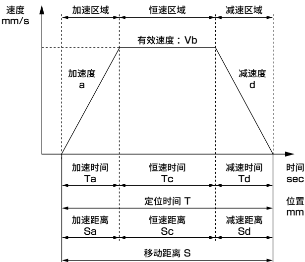
一般搬送动作的定位时间
