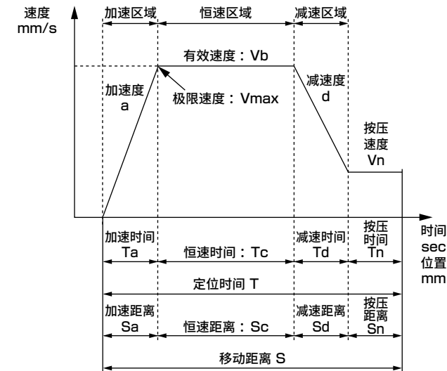
按压动作的定位时间
