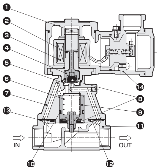
(图为打开动作时)
