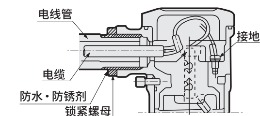
〈电线管螺纹时〉
