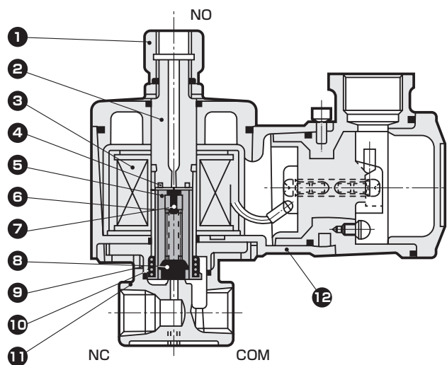
图示为AG41・43・44E4。
